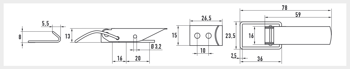
Nietloch / rivet hole / trou pour rivet Ø 3,35 mm / Ø 4,2 mm (Standard)
